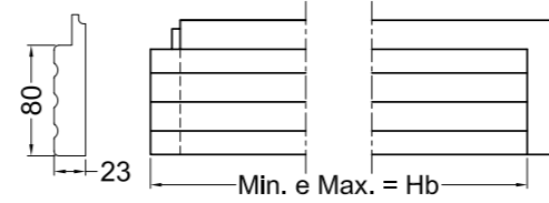
X2d - Angolo "interno" Inner corner | Angle interne | Ángulo interno Innenwinkel | Внутренний угол
