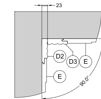
X2c - Angolo "interno" Inner corner | Angle interne | Ángulo interno Innenwinkel | Внутренний угол
