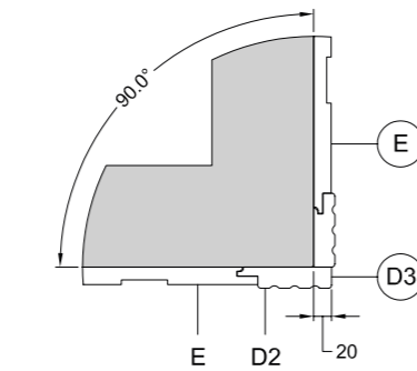
X2a - Angolo "esterno" Outer corner | Angle externe | Ángulo externo Aussenwinkel | Наружный угол
