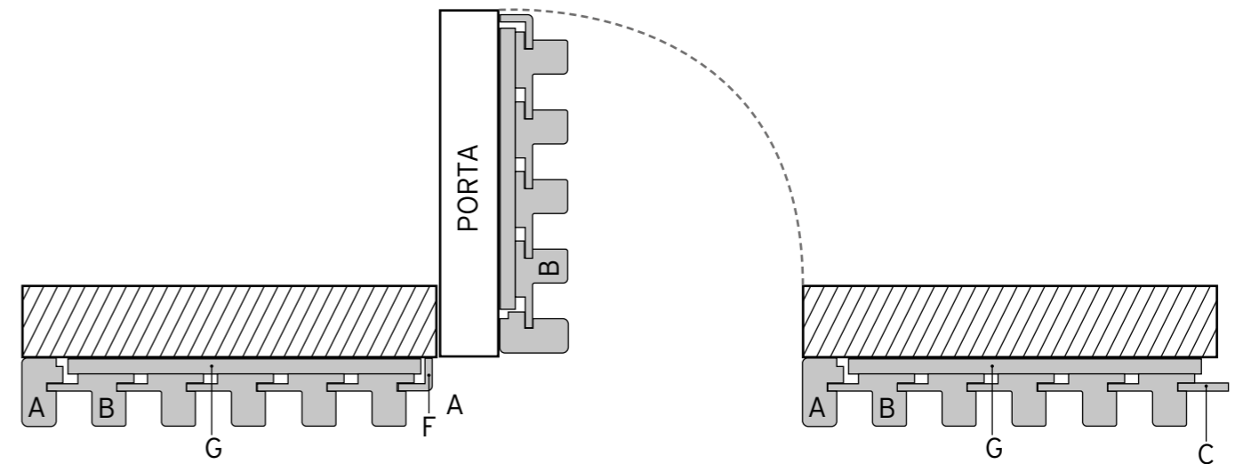
PARETE DRITTA CON PORTA | STRAIGHT WALL WITH DOOR | MUR DROIT AVEC PORTE | PARED RECTA CON PUERTA | GERADE WAND MIT TÜR | ПРЯМАЯ СТЕНА С ДВЕРЬЮ
