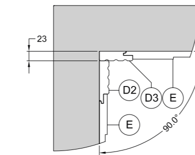
X2d - Angolo "interno" Inner corner | Angle interne | Ángulo interno Innenwinkel | Внутренний угол
