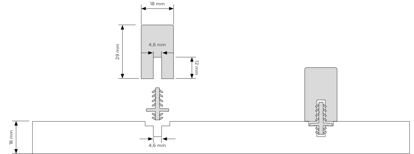
PANNELLO BOISERIE FISSATA A MURO | WALL-MOUNTED PANEL | PANNEAU BOISERIE FIXÉE AU MUR PANEL DE BOISERIE FIJADO EN PARED | AN DER WAND BEFESTIGTE TÄFELUNGSPLETTE | ПАНЕЛЬ, ПРИКРЕПЛЕННАЯ К СТЕНЕ
