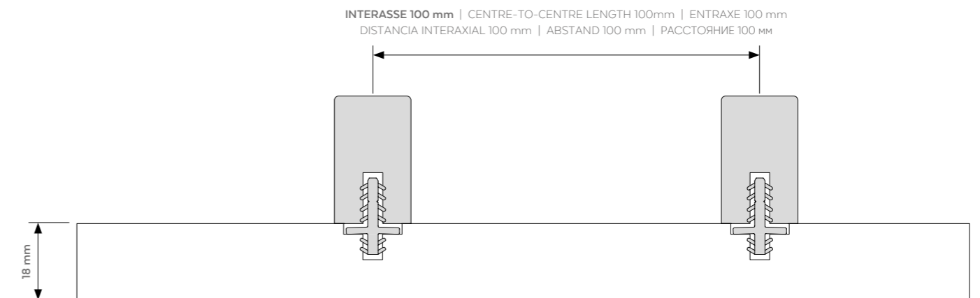
PANNELLO BOISERIE FISSATA A MURO | WALL-MOUNTED PANEL | PANNEAU BOISERIE FIXÉE AU MUR PANEL DE BOISERIE FIJADO EN PARED | AN DER WAND BEFESTIGTE TÄFELUNGSPLETTE | ПАНЕЛЬ, ПРИКРЕПЛЕННАЯ К СТЕНЕ
