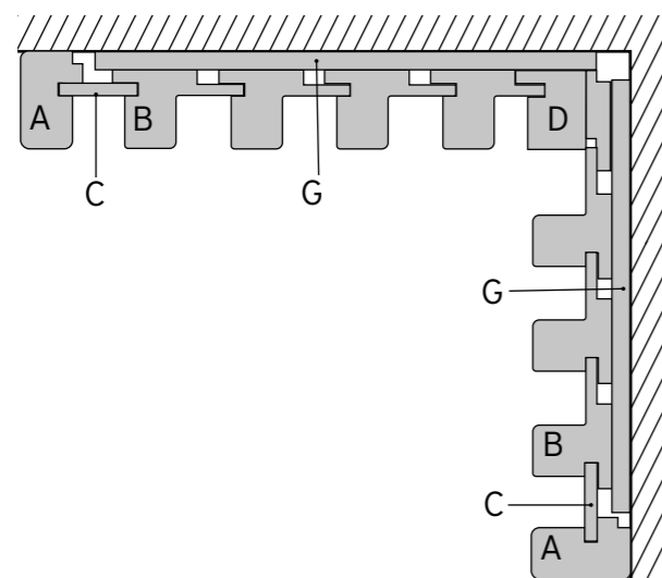
PARETE ANGOLO INTERNO | INTERIOR CORNER WALL | MUR D'ANGLE INTÉRIEUR | PARED ÁNGULO INTERNO | WAND MIT INNENWINKEL | ВНУТРЕННИЙ УГОЛ СТЕНЫ
