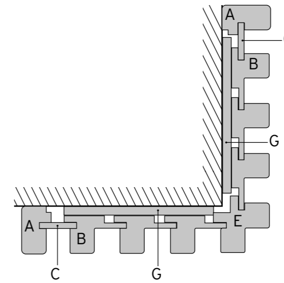
PARETE ANGOLO ESTERNO | EXTERNAL CORNER WALL | MUR D'ANGLE EXTÉRIEUR | PARED ÁNGULO EXTERNO | WAND MIT AUSSENWINKEL | ВНЕШНИЙ УГОЛ СТЕНЫ
