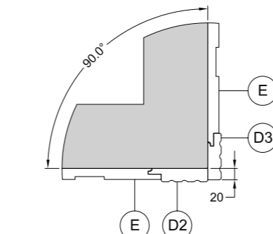
X2b - Angolo "esterno" Outer corner | Angle externe | Ángulo externo Aussenwinkel | Наружный угол
