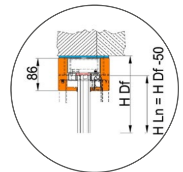
DETTAGLIO LATERALE LATERAL DETAIL
