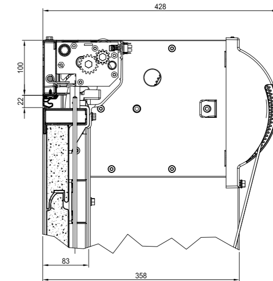
SEZIONE VERTICALE VERTICAL SECTION
