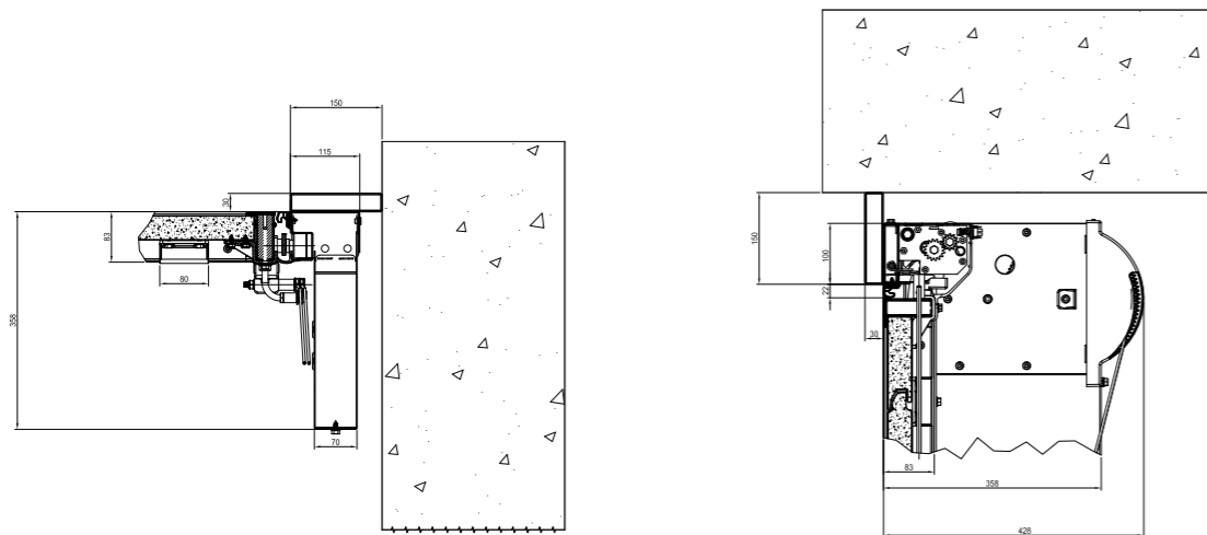
SEZIONE VERTICALE VERTICAL SECTION
