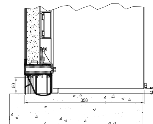
Dettaglio soglia per porta senza portina pedonale Threshold detail for door without pedestrian door
